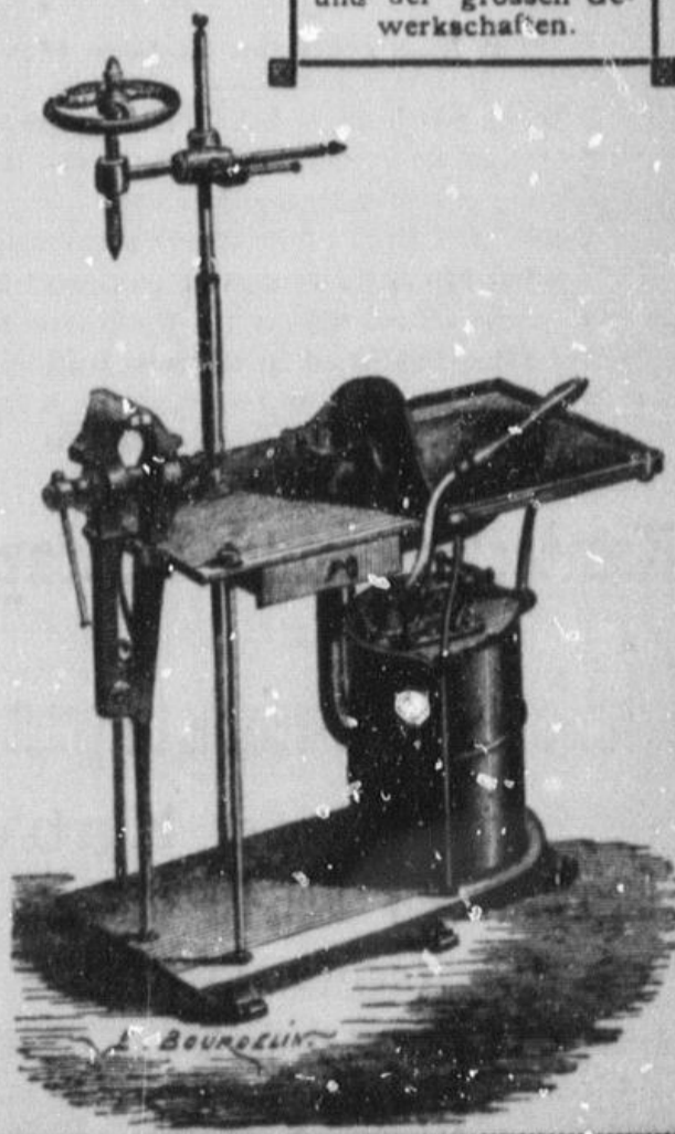
Tragbare Schmiede, mit doppeltem Gebläse u. drehbarem Hebel.
