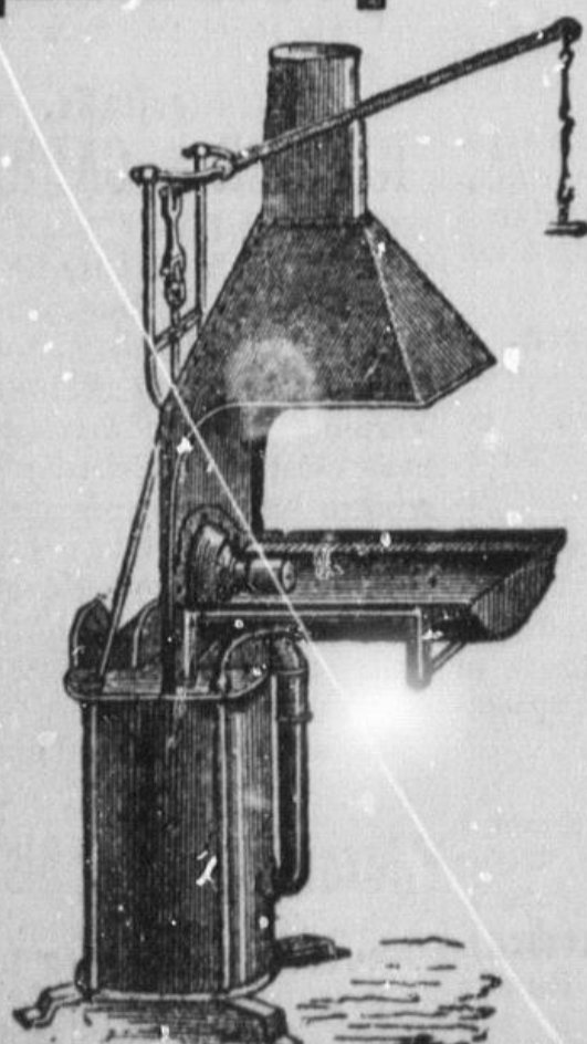
Tragbare Schmiede, mit doppeltem Gebläse u. drehbarem Hebel.
