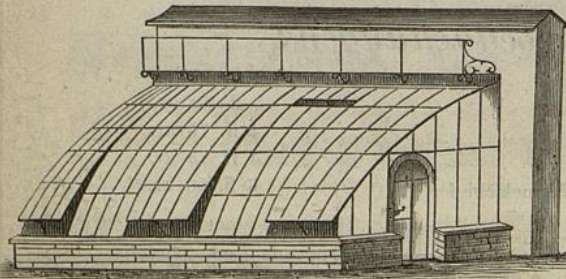
Anlehnendes Treibhaus
