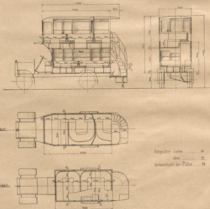
Abb. 249. Kraft-Stellwagen mit geschlossenem Obergeschoß, Wiener Typ (Patent Spängler)
