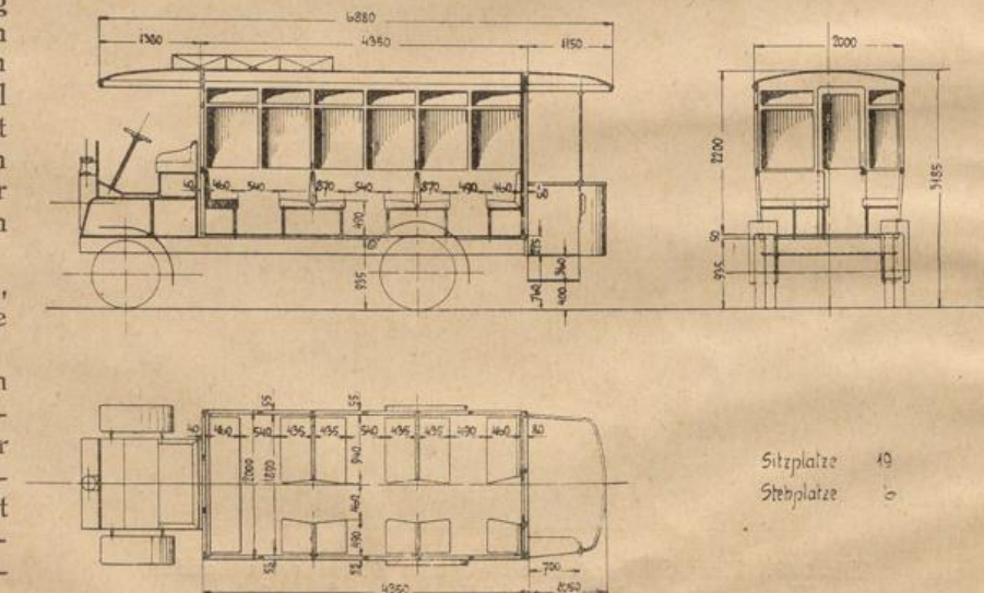
Abb. 245. Eingeschossiger Kraft-Stellwagen, Pariser Typ. (Chassis von De Dion-Bouton)
