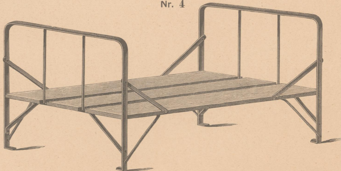
Cavalette Nr. 4, braun gestrichen, aus massivem Flacheisen, mit Holzeinlagen, Kopf- und Fusstheile sind zum Zusammenklappen, so dass die ganze Länge des Cavalettes in zusammengeklapptem Zustande der Länge der Holzeinlagen gleich ist
