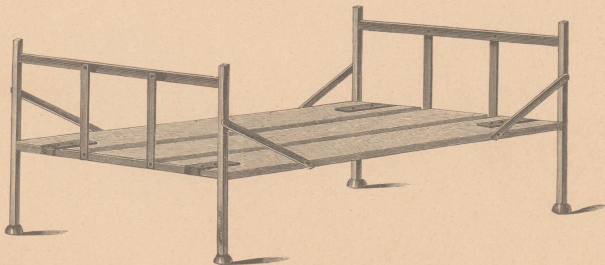
Cavalette Nr. 3 (ärarische Form), aus massivem □Eisen, braun gestrichen, die Füße mit gepressten Scheiben, sogenannten Glocken versehen, mit Holzeinlagen
