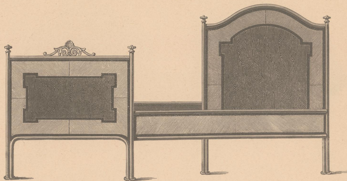
Bett Nr. 55 zweifärbig nussartig lackirt 80 cm breit, 182 cm lang fl. 22.50 95 cm „ 190 cm „ „ 24.25 schwarz oder nussartig lackirt, vergoldet und bemalt 80 cm breit, 182 cm lang fl. 25.50 95 cm „ 190 cm „ „ 27.25
