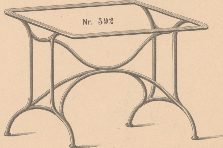
Tischgestelle Nr. 592 für Platten breit 47—50 60—65 cm lang 70—75 95—100 cm
