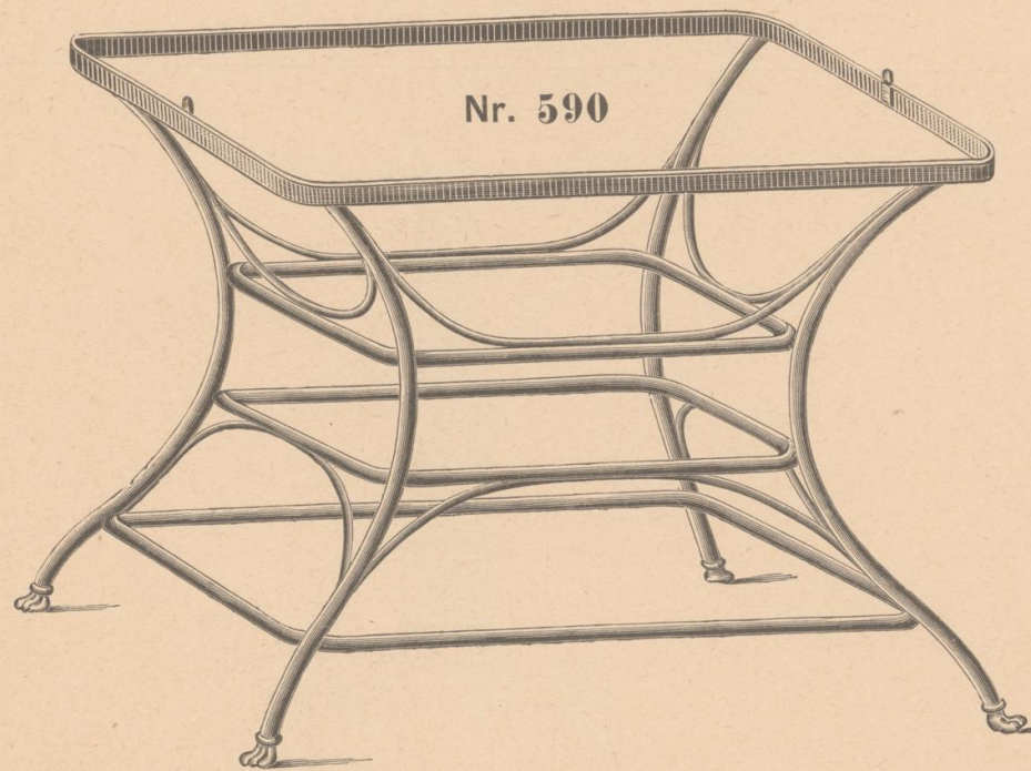
Tischgestelle Nr. 590 für Platten breit 47—50 60—65 70—75 cm lang 70—75 95—100 115—125 cm
