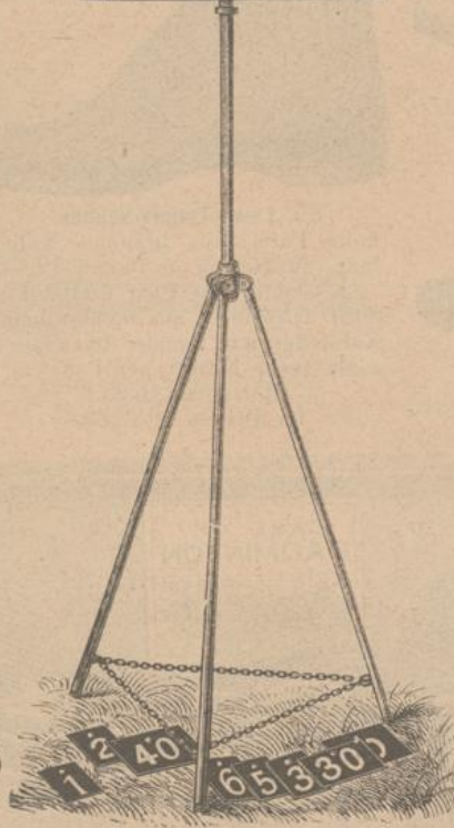
88. Markirtafel auf zusammenlegbarem Eisenständer mit auswechselbaren Blechnummern fl. 15.—.
