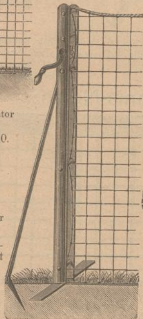
1562. Lawn-Tennis-Netzständer „Climax“ mit praktischer Spannvorrichtung und starkem, doch leichtem Eisenfuss, für Gras- und Sandplätze sehr zu empfehlen, ausserordentlich standhaft, per Paar fl. 26.50.
