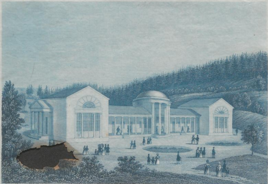
DER FERDINANDSBRUNN.
