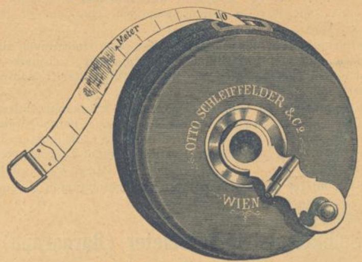
Fig. 61. Messband in Lederkapsel, 20 Meter lang, in 1/2 der natürlichen Grösse.
