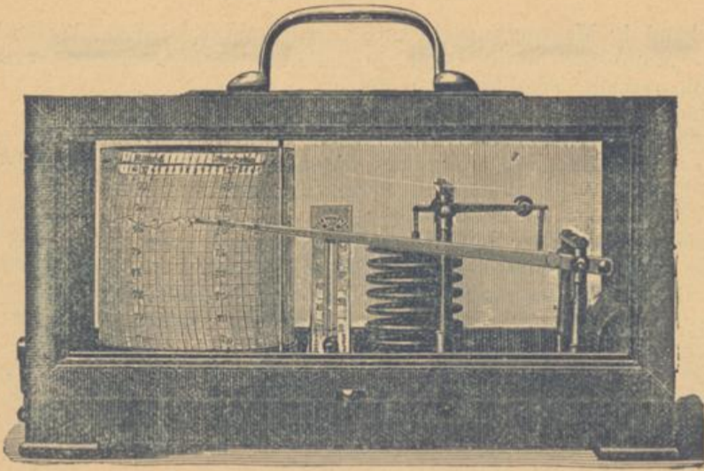
Fig. 49. Selbstregistrier-Barometer in 1/3 der natürlichen Grösse.
