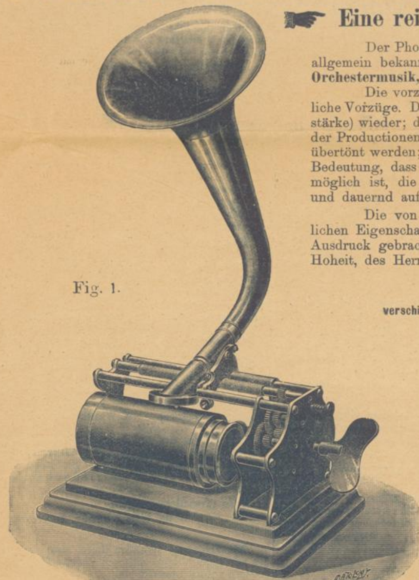
Amerikanischer Phonograph Nr. 1, 1/4 der natürlichen Grösse.
