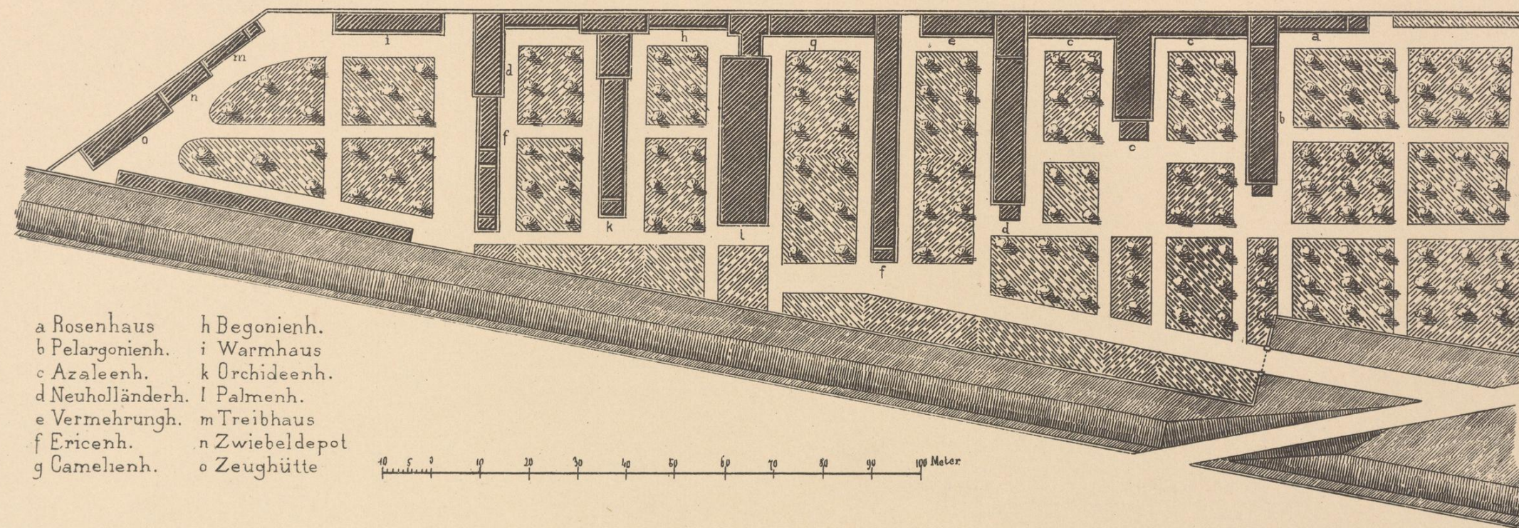
GRUNDRISS.
