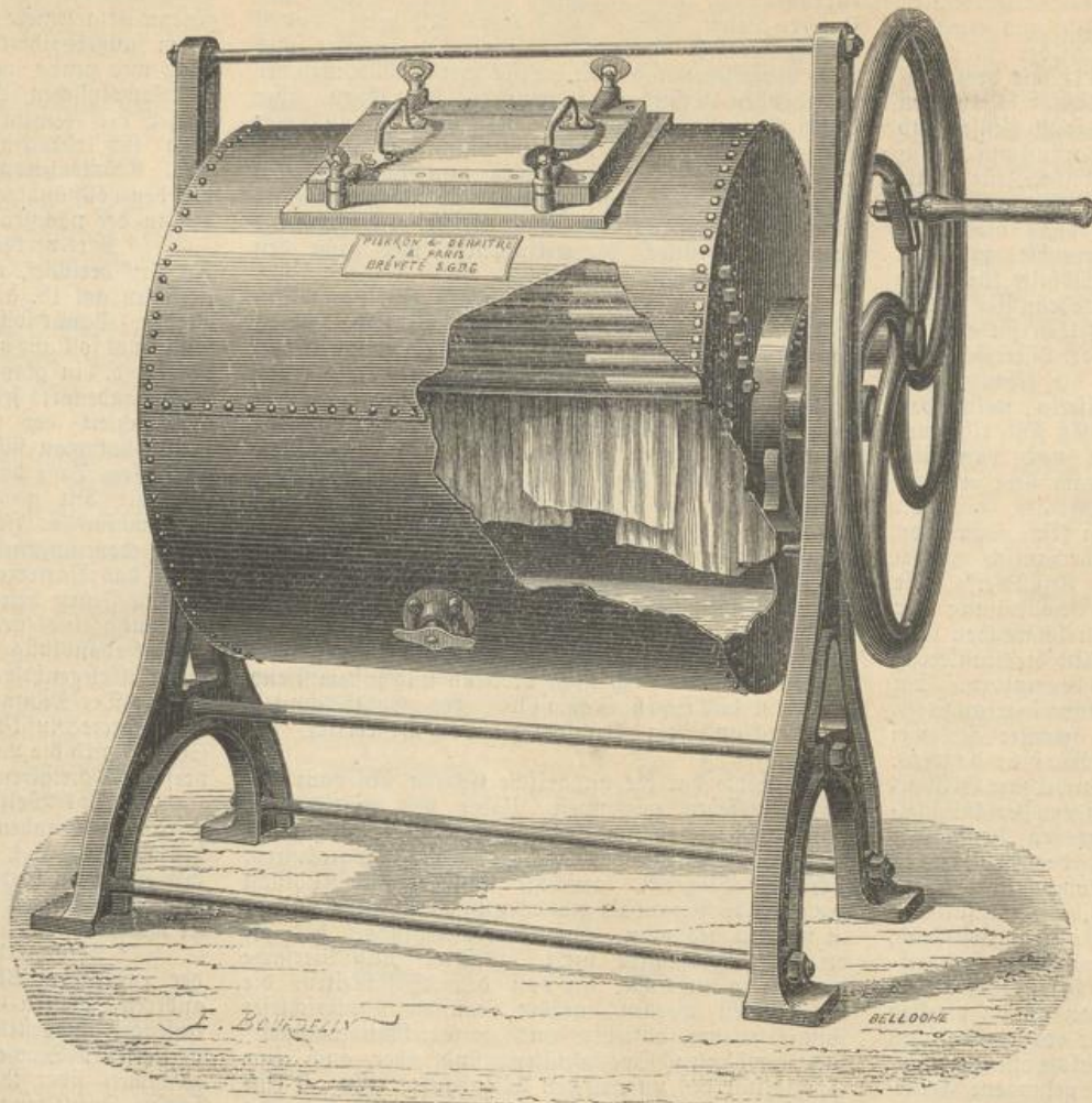
Washmaschine von Pierron & Dehaitre in Paris.
