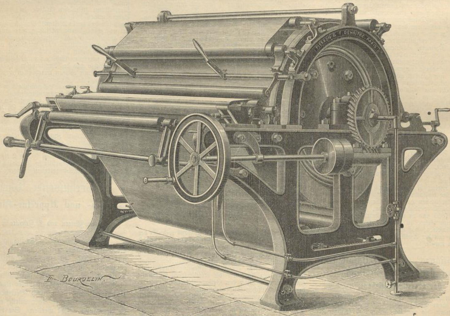
Appreturmaschine von Pierron & Dehaitre in Paris.
