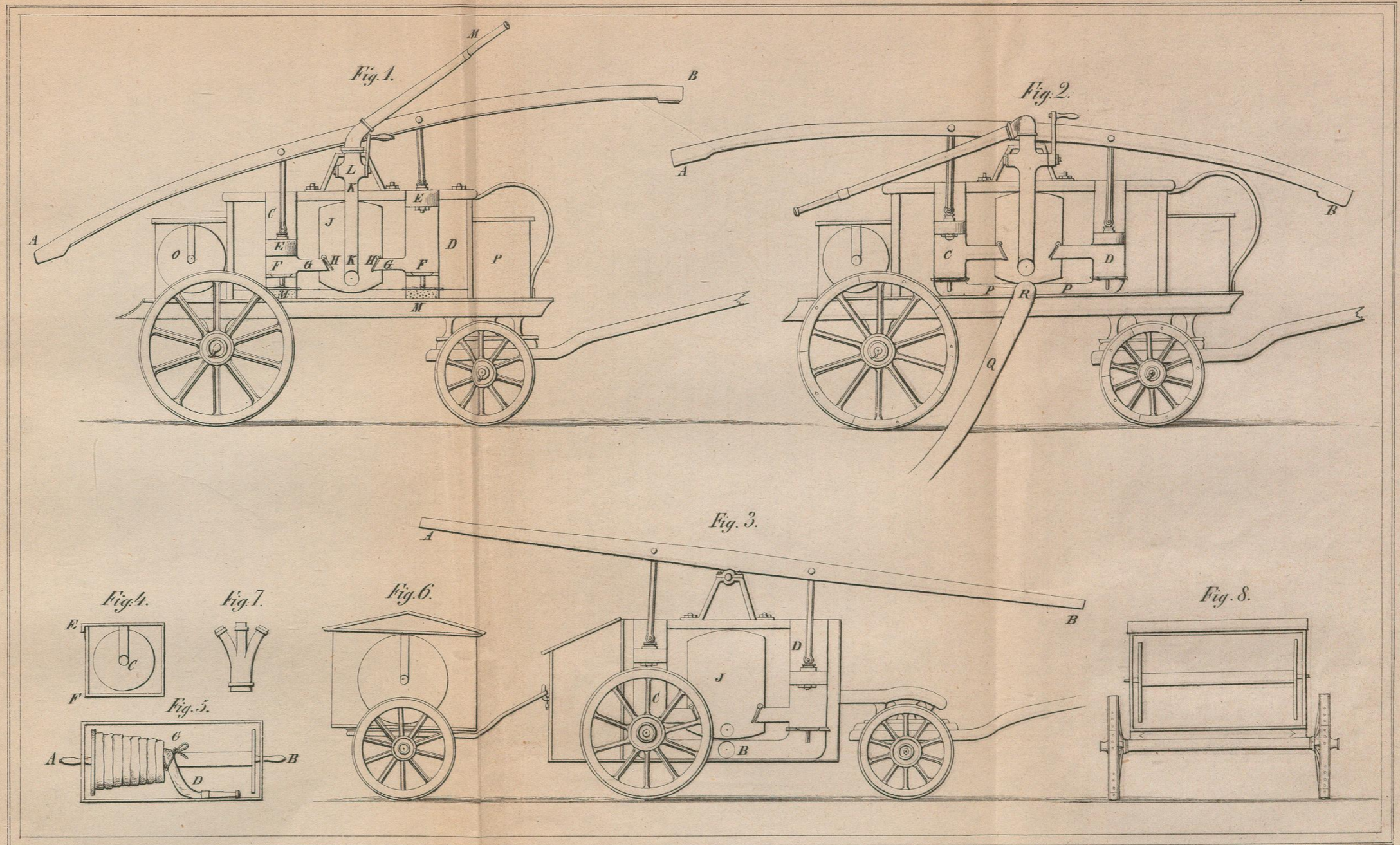
GROSSE FAHRSPRITZE — SPRITZE MIT SAUGWERK — WASSERZUBRINGER — SCHLAUCHHASPEL.
